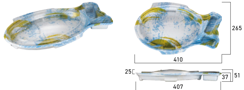
DRE-SASHIMI-16-4 DRE-회16-4 Patent No : 30-2022-0031186 410×265×51(SET)
